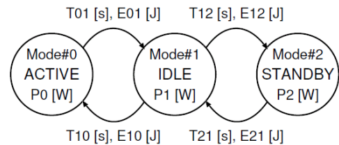
図1 典型的な3モードディスクドライブの消費電力の状態遷移モデル
