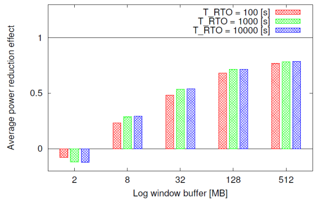
図2 ディスクストレージの省電力化効果 (TPC-C) Fig.2 Power reduction effect on disk storage (TPC-C).
