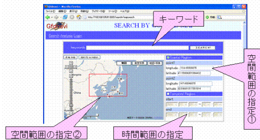
図 5 検索インタフェース
