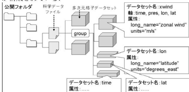
図2 一般的な地球科学データファイルの構造
