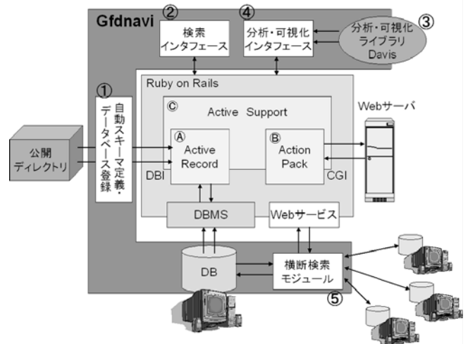
図1 Gfdnavi の構成
