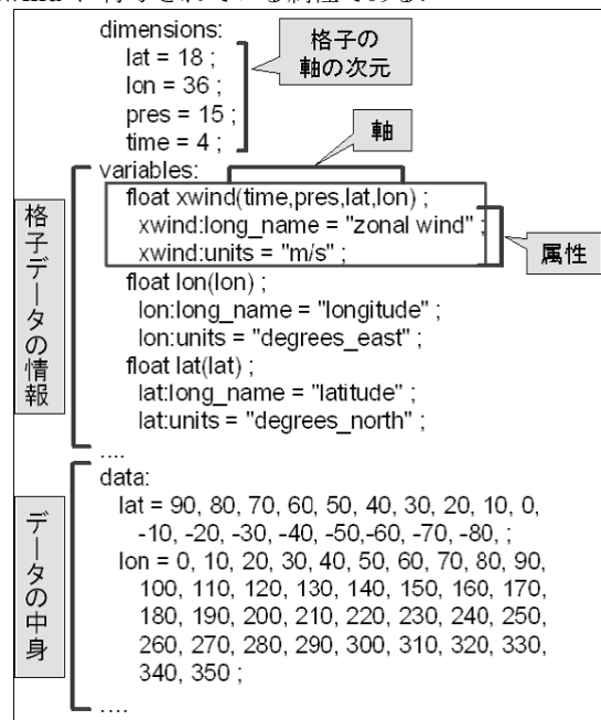
図3 NetCDF のヘッダ情報例
